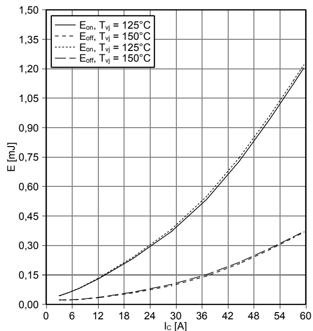
Schaltverluste MOSFET (typisch) switching losses MOSFET (typical)
